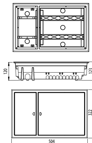
09QI2X15-D Quadro interior para 30 módulos + Diferencial
